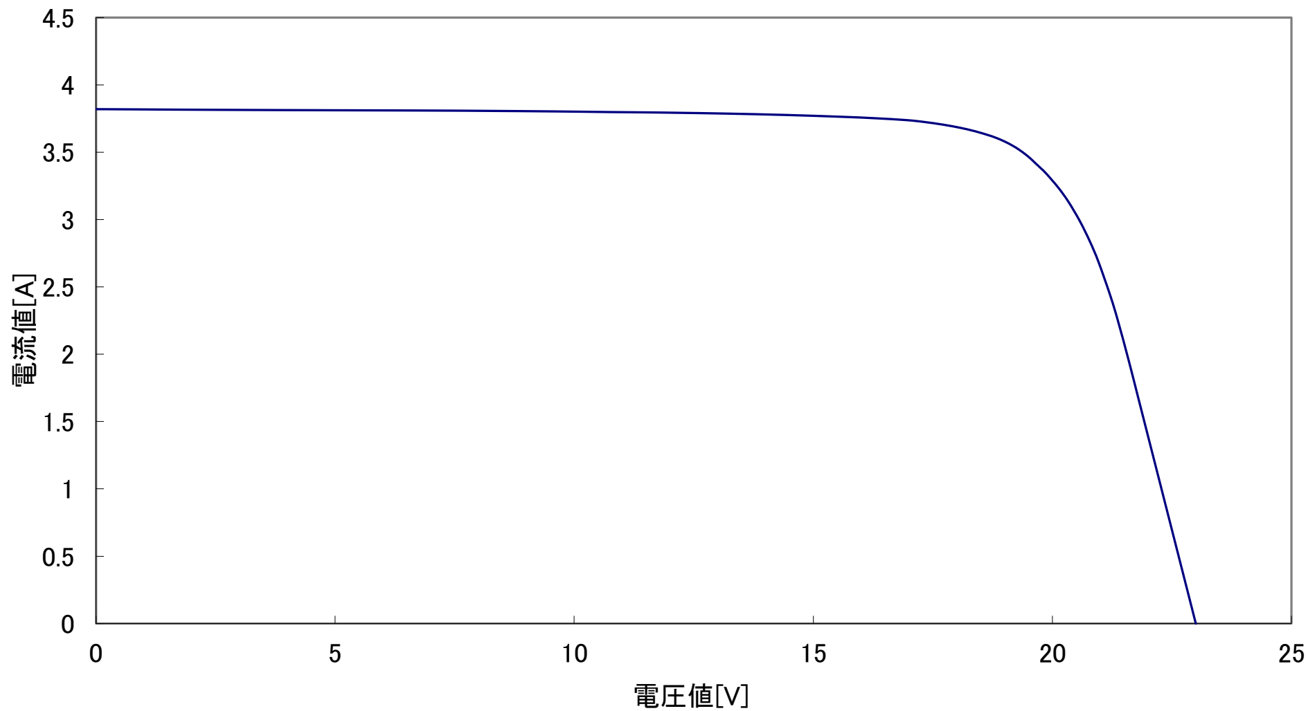
GN68R 出力特性図 @1000W/m 2 AM1.5 25°C
