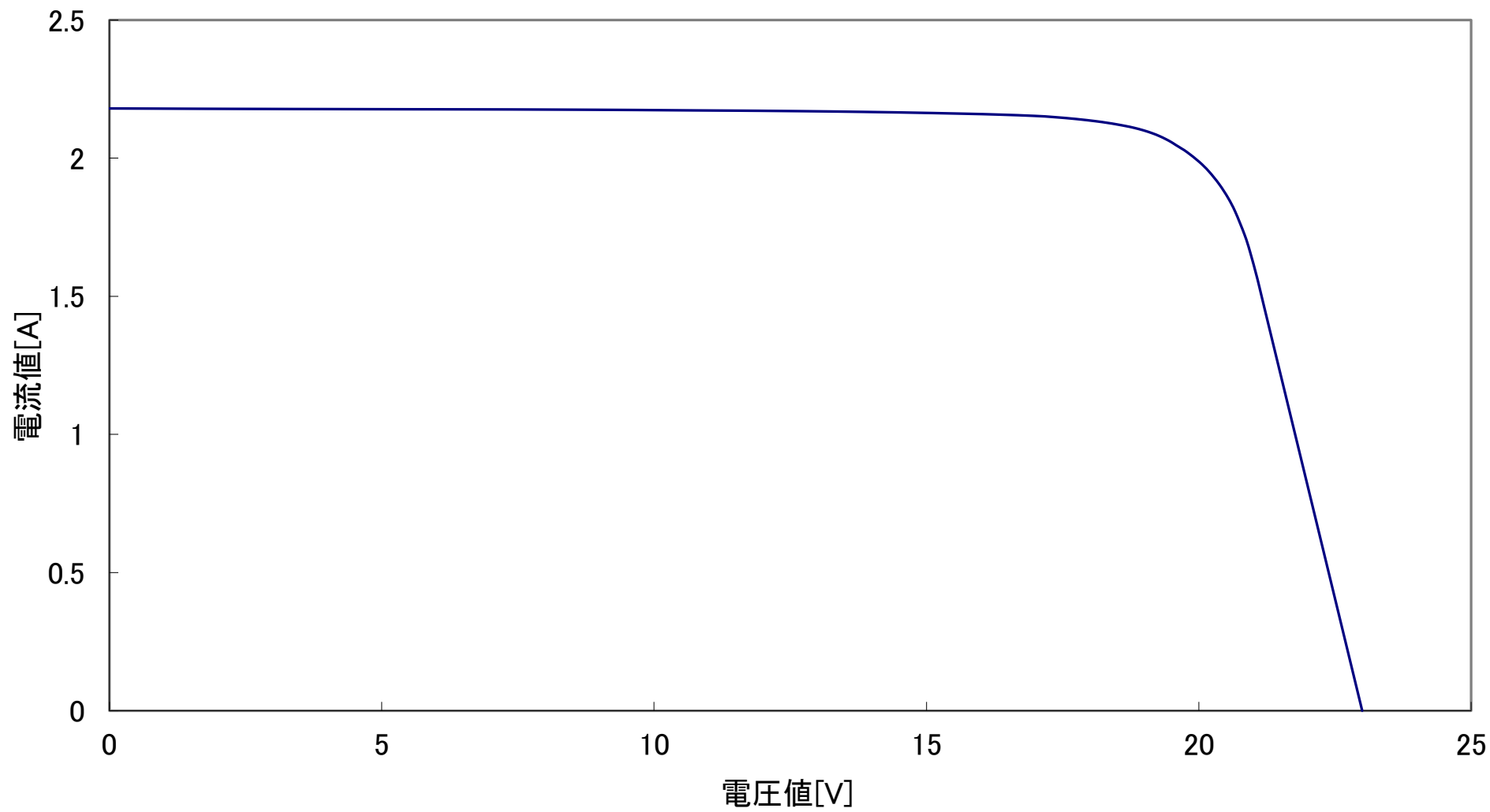
GN40R 出力特性図 @1000W/m 2 AM1.5 25°C
