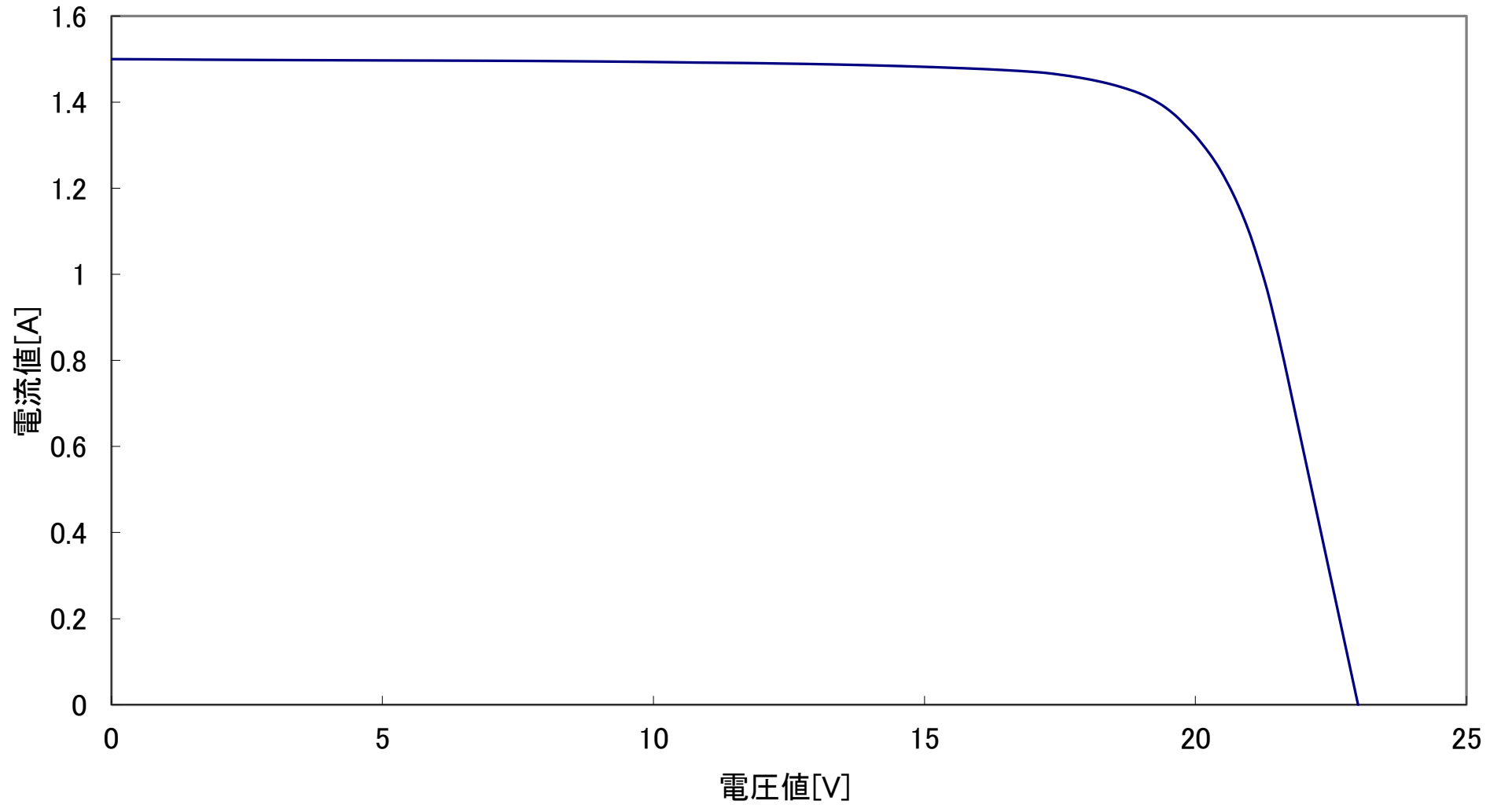
GN27R 出力特性図 @1000W/m 2 AM1.5 25°C
