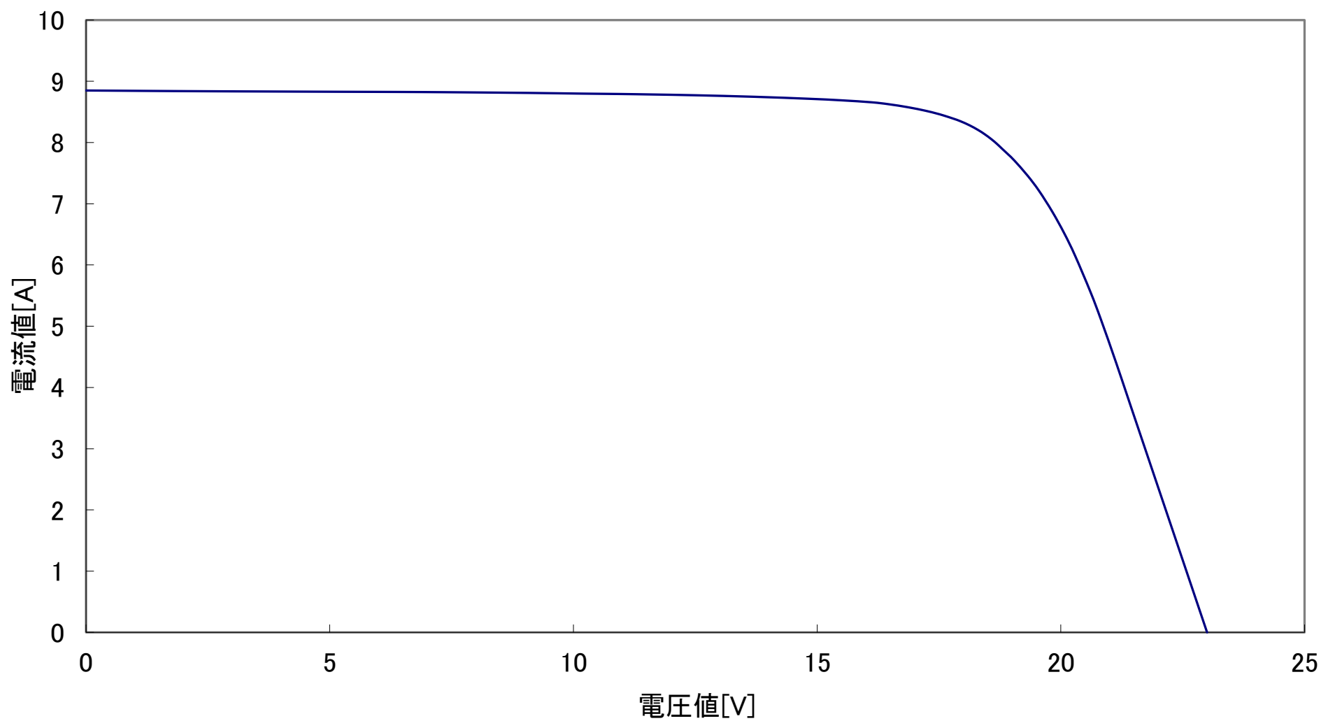
GN150R 出力特性図 @1000W/m 2 AM1.5 25°C
