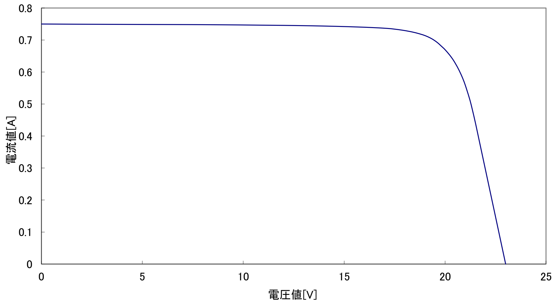
GN13R 出力特性図 @1000W/m 2 AM1.5 25°C
