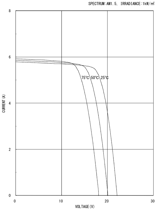
太陽電池モジュールKD95SX-RPの電流-電圧特性の温度依存性
