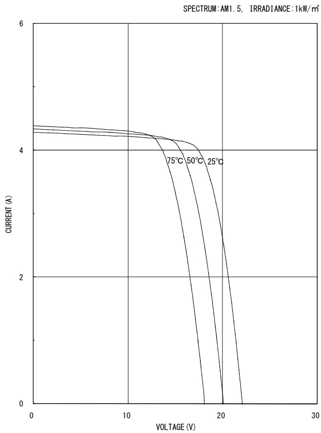
太陽電池モジュールKD70SX-RPの電流-電圧特性の温度依存性
