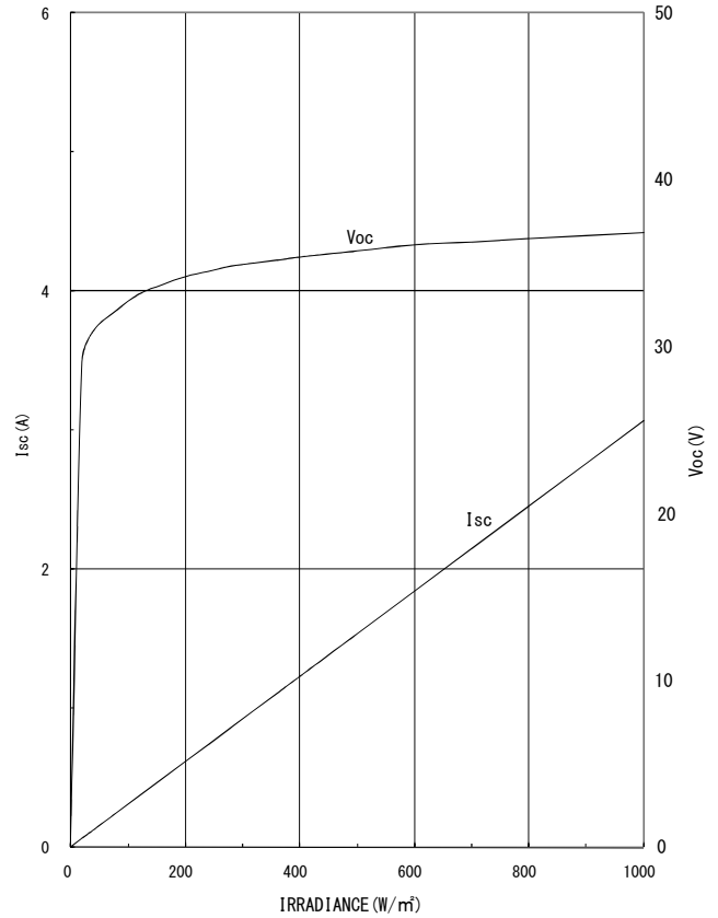
太陽電池モジュールKD50SE-RPの短絡電流、開放電圧の照度依存性
