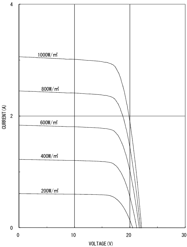
太陽電池モジュールKD50SE-RPの電流-電圧特性の照度依存性
