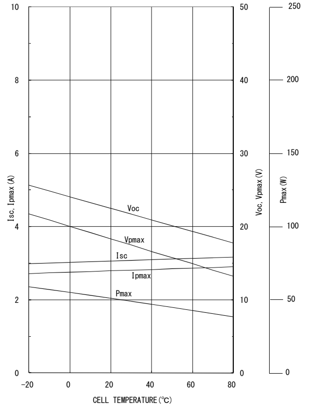
太陽電池モジュールKD50SE-RPの最大出力、開放電圧、短絡電流、最大出力動作電圧、最大出力動作電流の温度依存性
