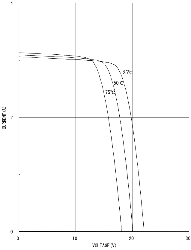
太陽電池モジュールKD50SE-RPの電流-電圧特性の温度依存性
