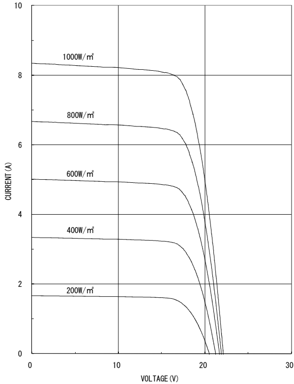
太陽電池モジュールKD135SX-RPの電流-電圧特性の照度依存性
