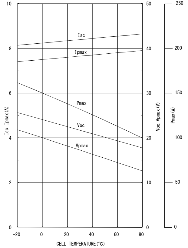
太陽電池モジュールKD135SX-RPの最大出力、開放電圧、短絡電流、最大出力動作電圧、最大出力動作電流の温度依存性
