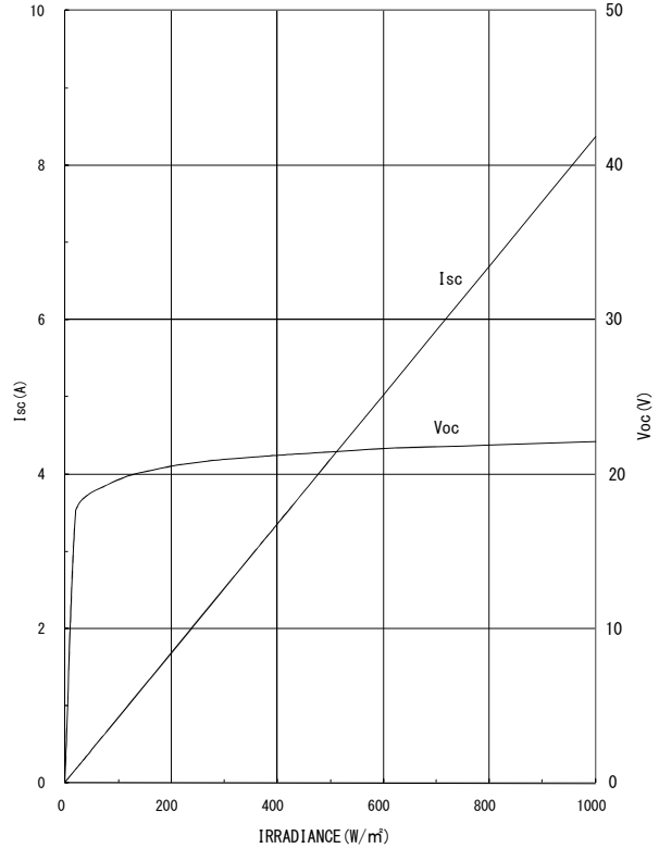
太陽電池モジュールKD135SX-RPの短絡電流、開放電圧の照度依存性
