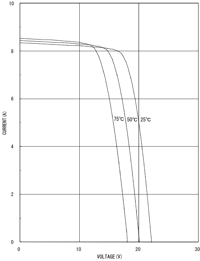
太陽電池モジュールKD135SX-RPの電流-電圧特性の温度依存性
