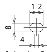
長丸穴詳細図
