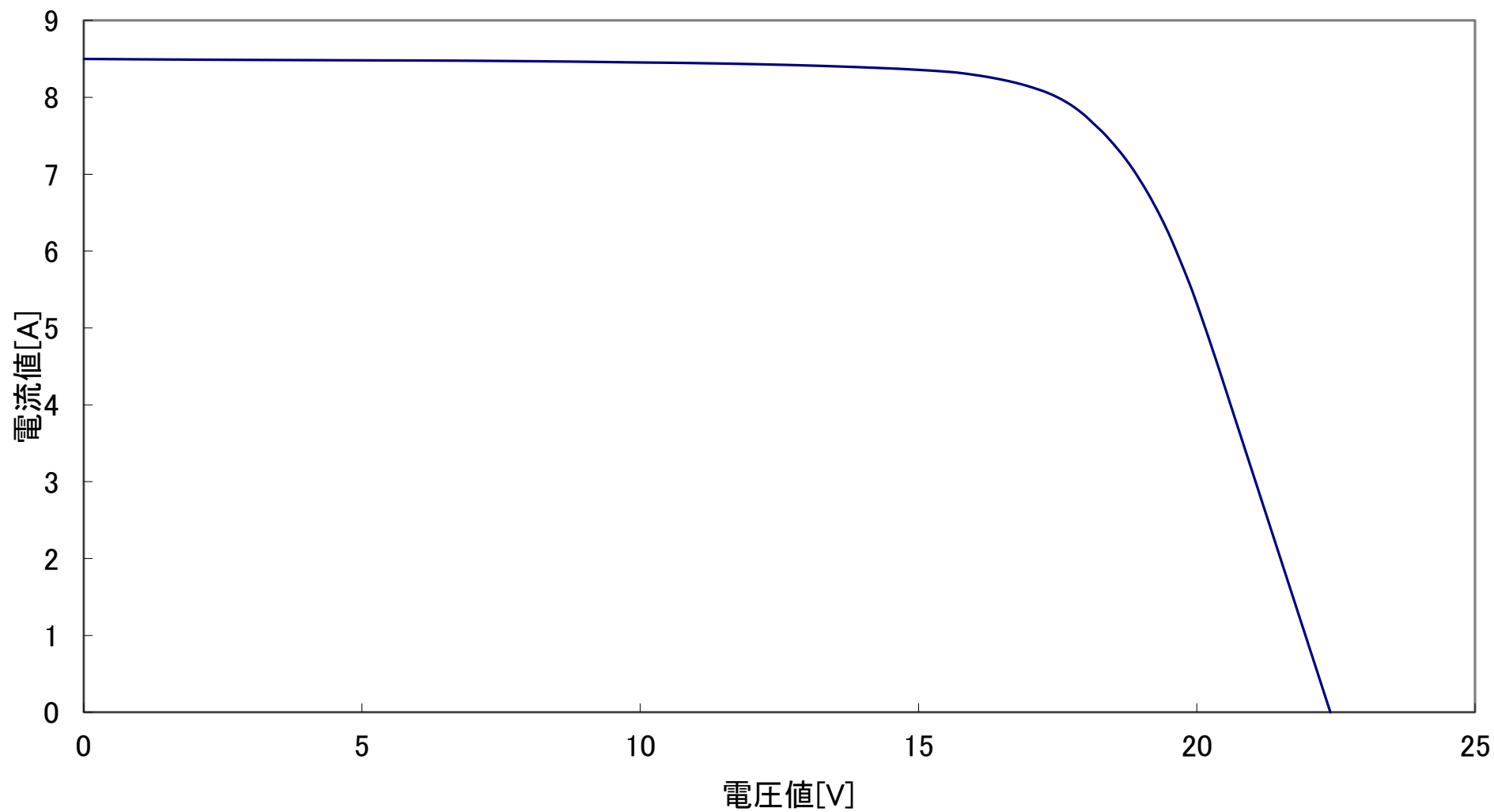
GN140 出力特性図 @1000W/m 2 AM1.5 25°C
